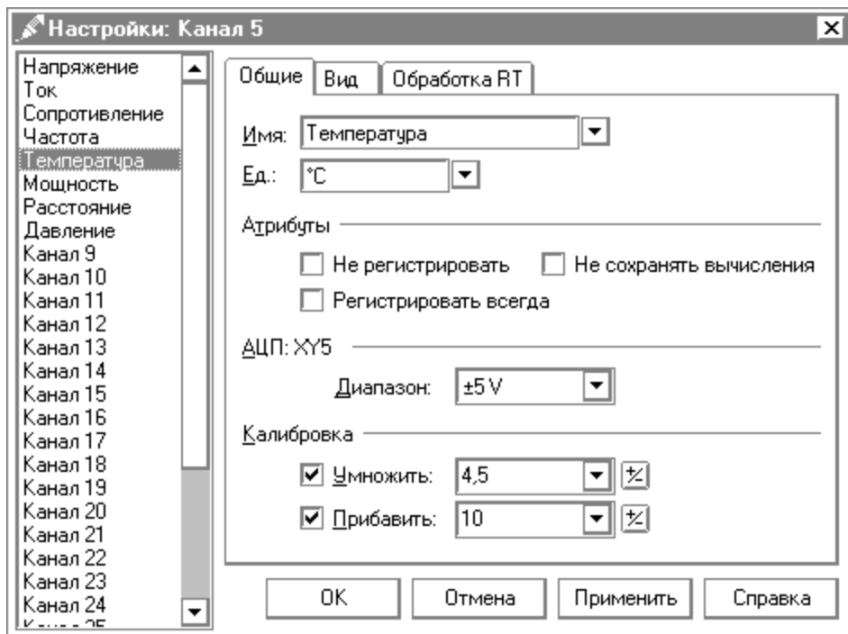
Рис.2.2. Окно свойств канала. Общие настройки.
