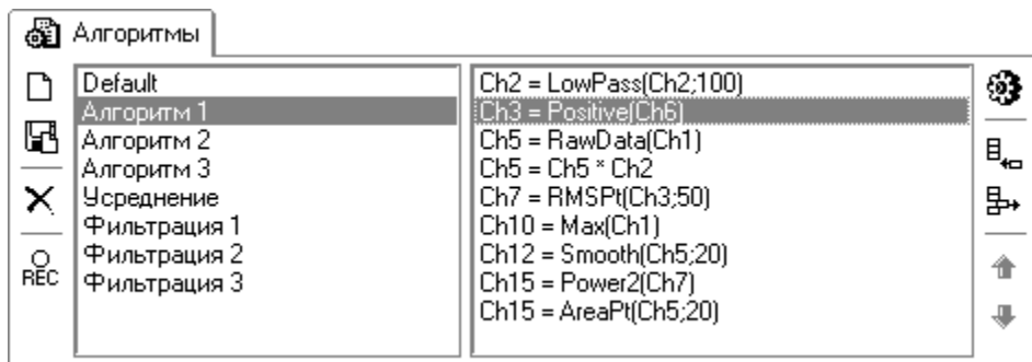
Рис. 7.2. Вкладка "Алгоритмы".
