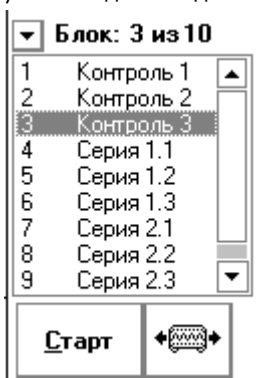
Рис. 6.1. Панель записи.
