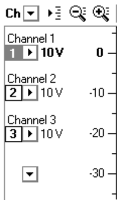
Рис. 2.1. Шкала амплитуды
