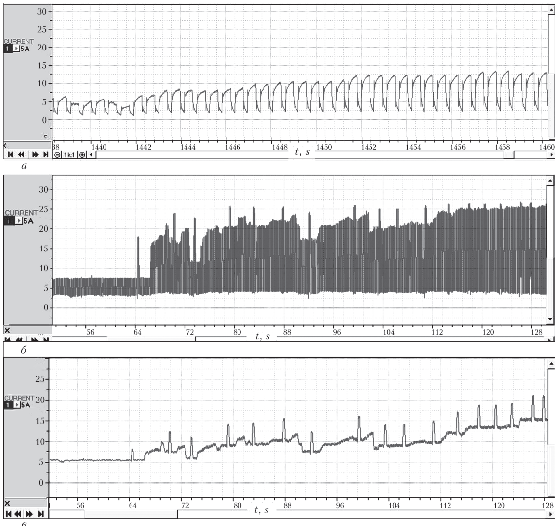
Рис. 4. Внешний вид фрагментов циклограммы режима микроплазменной порошковой наплавки I(t) = U_{c1}(t)K_I после первичной цифровой обработки, частота регистрации сигнала 2,5 кГц: а — стабилизированный сварочный ток, установка STARWELD PTA 190H фирмы «Kennametal Stellite GmbH»; б, в — нестабилизированный сварочный ток, установка УПНС-304M2/M3, частота пульсаций сварочного тока 150 Гц
