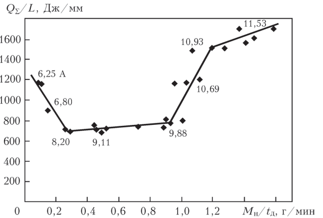
Рис. 6. Зависимость погонной энергии Q_{\Sigma}/L от производительности M_H/t_d и изменения средней величины сварочного тока при наплавке на узкую подложку шириной 1,6 мм
