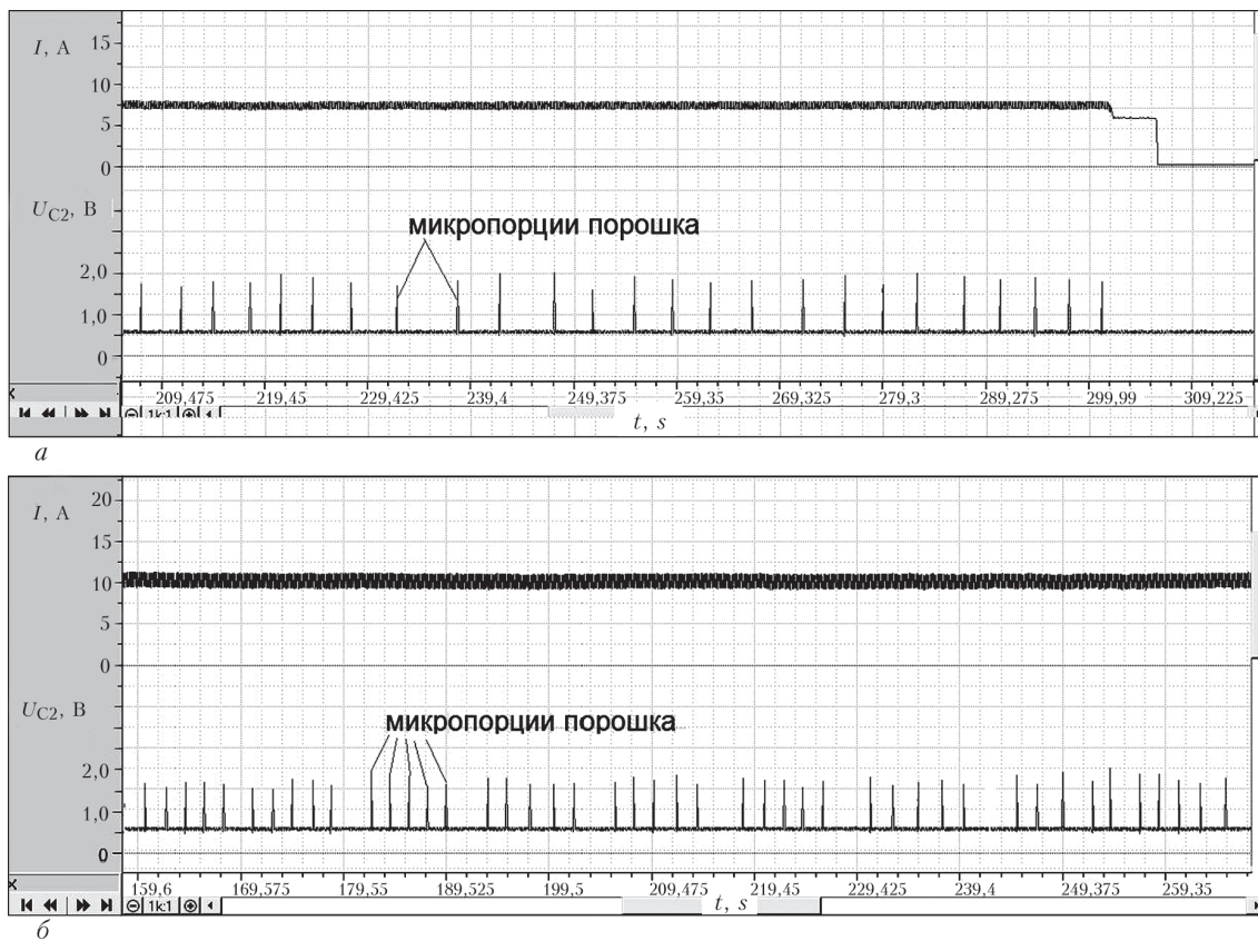
Рис. 5. Фрагменты осциллограмм микроплазменной порошковой наплавки на узкую подложку \delta = 1,6 мм с различным количеством микрорпорций дисперсной присадки, вводимой в сварочную ванну, шт.: а — 1; б — 5
